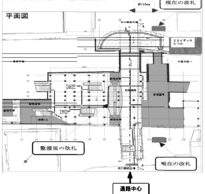
新小岩駅南北自由通路整備図
