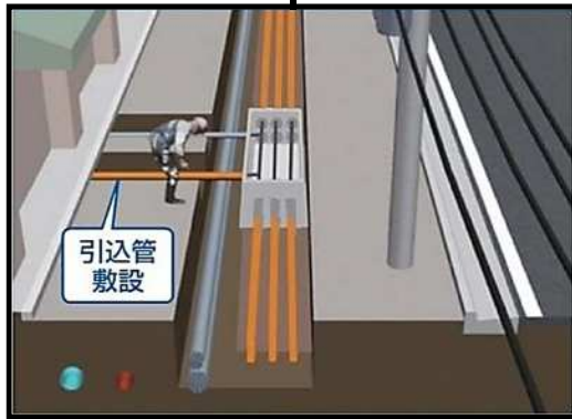
各家庭に電力や通信を供給するための管を埋設します。
